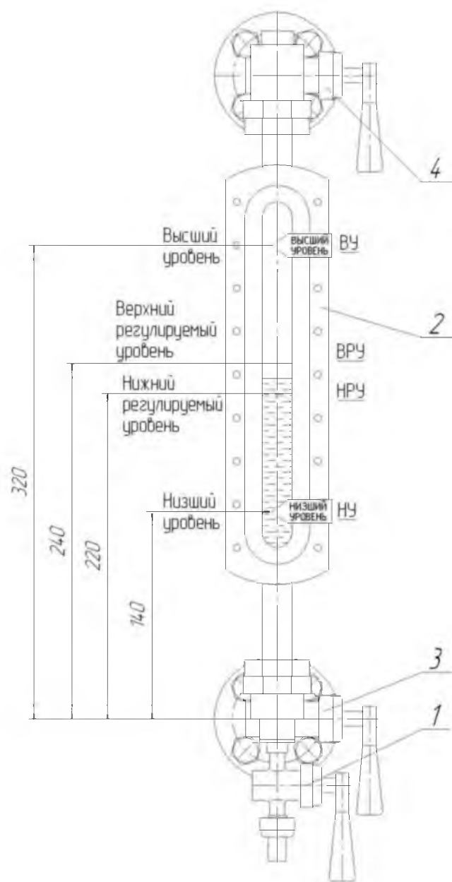
Рис.14 Водоказательный прибор 1-пробно-спускной кран; 2-рамка; 3-нижний кран; 4-верхний кран.
