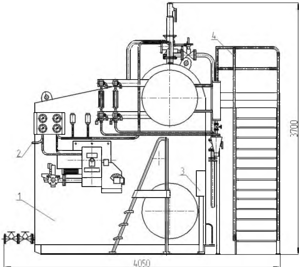
Рис. 1 Котёл паровой Е-4.0-1.4 ГМ
