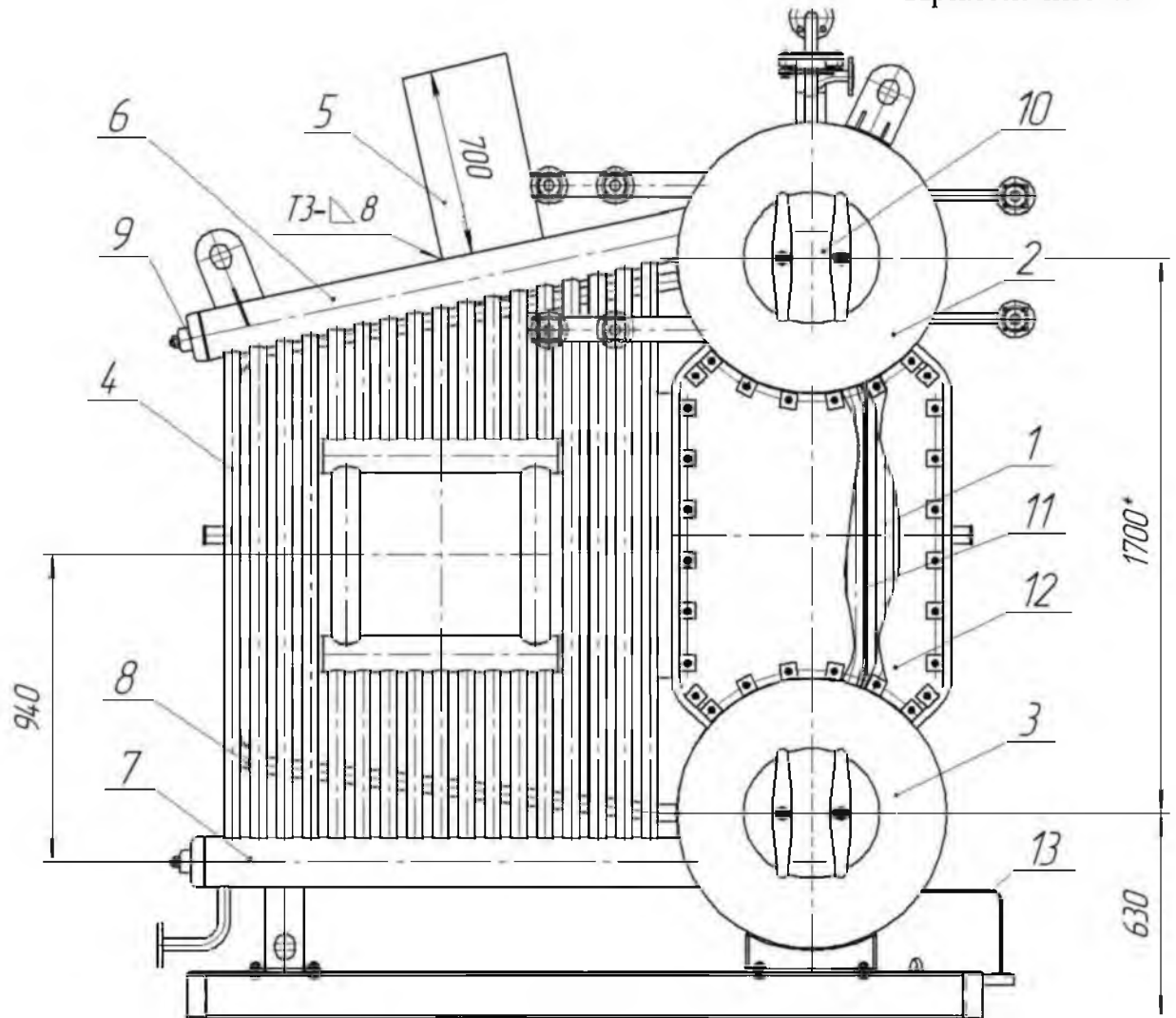
Рис. 2 Система трубная.
