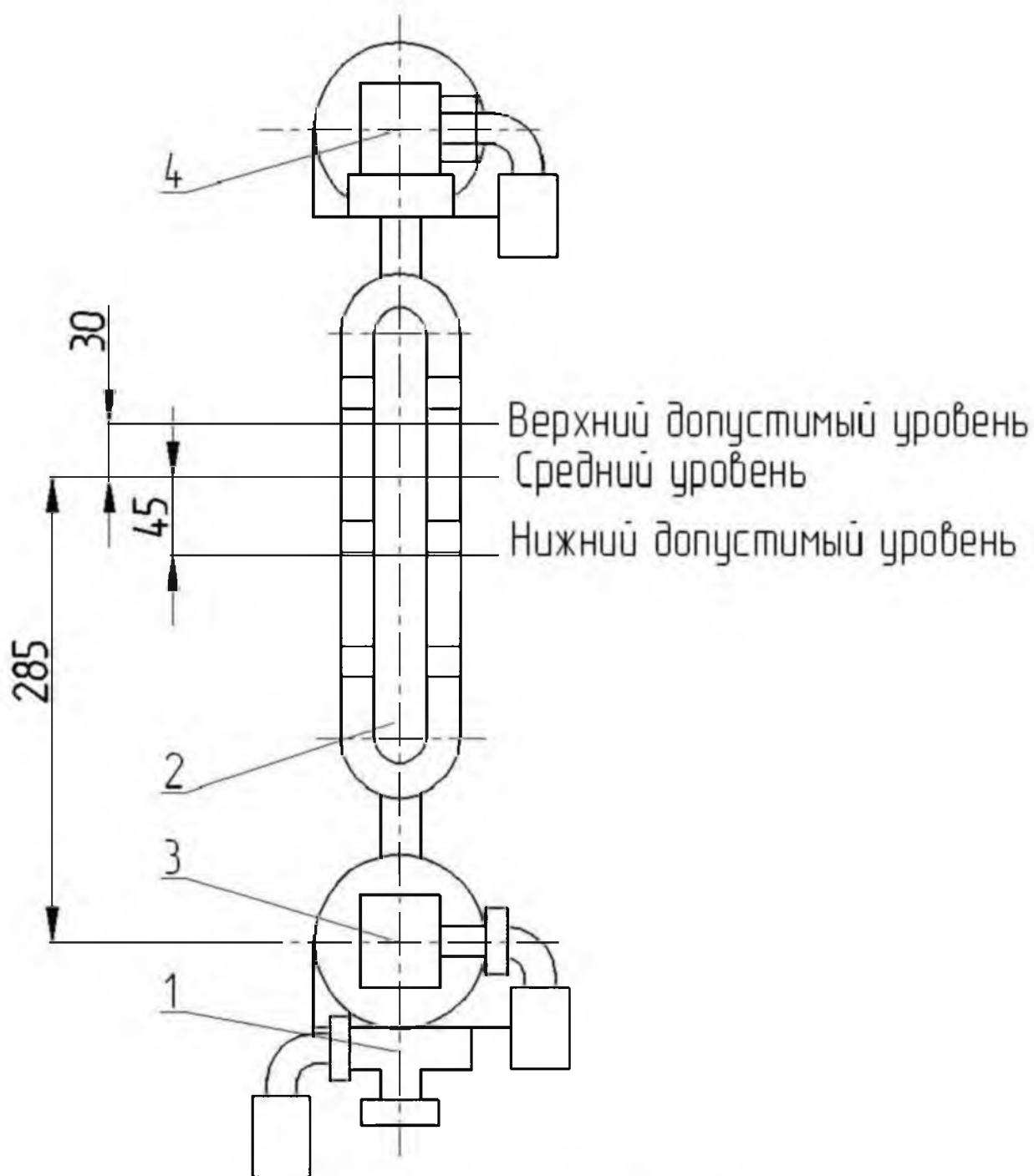
Рис. 3 Водоуказательный прибор.
