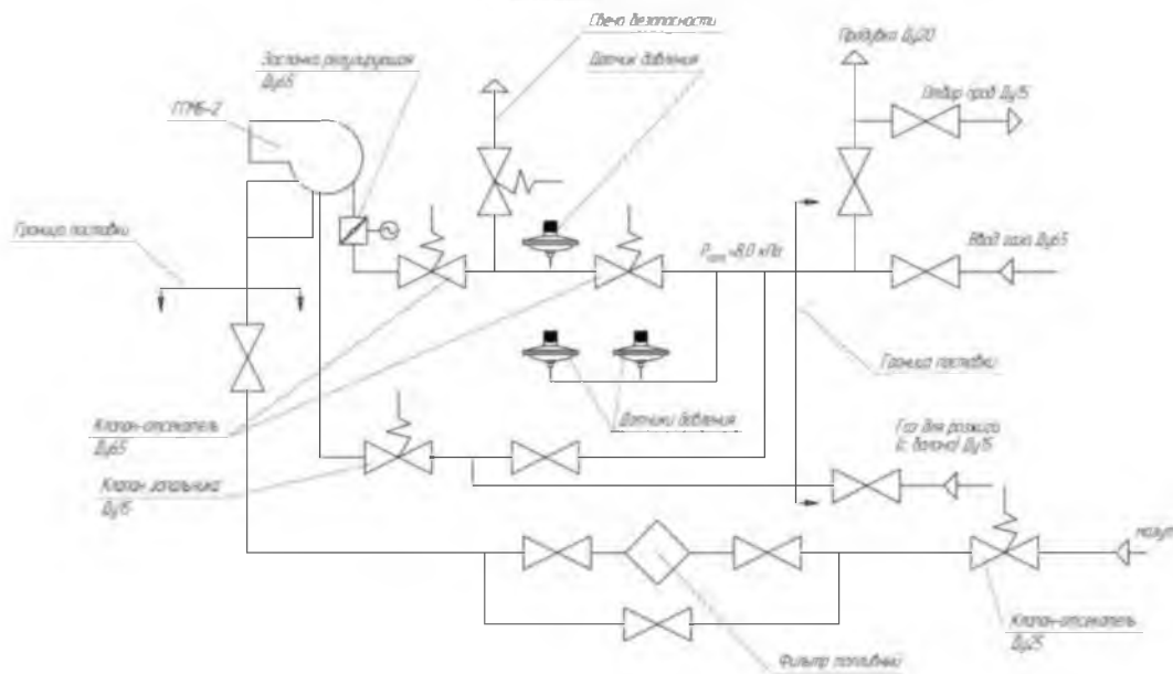
Принципиальная схема подачи газа к котлу с горелкой ПТМБ-2
