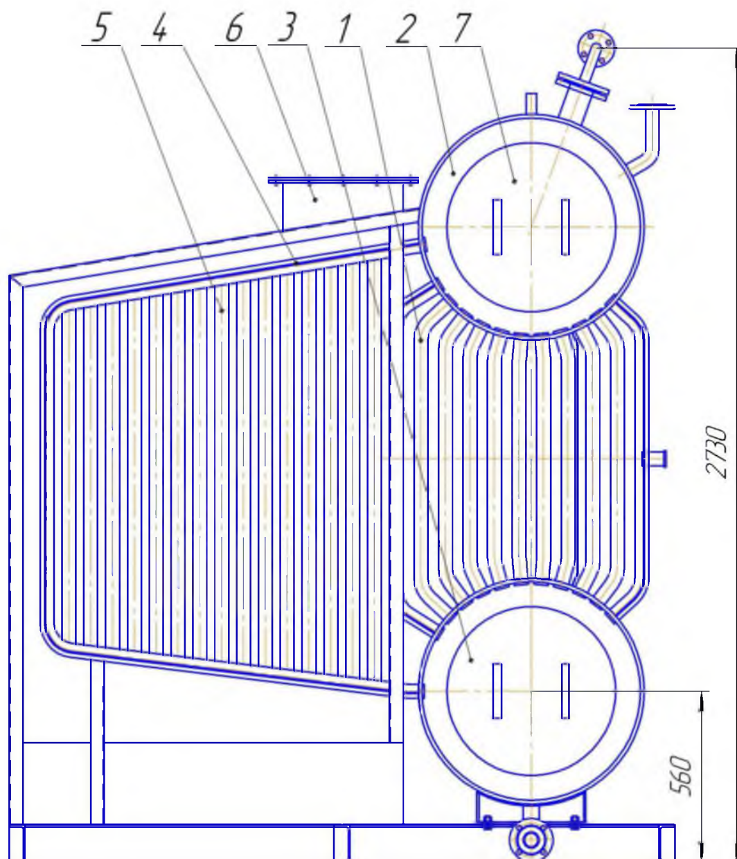
Рис 2 Система трубная
