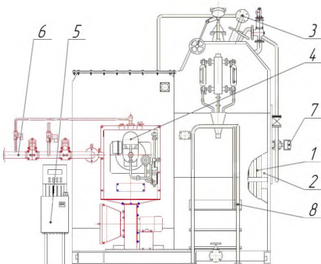
Рис.1 Котел паровой
