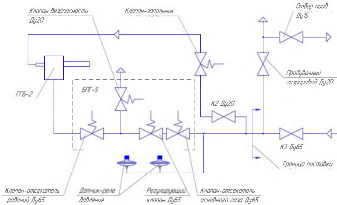
Принципиальная схема подачи газа к котлу с горелкой ГГБ-2 (позиционное регулирование) Е-1,6-09ГМН - P_{газа} = 4,0 кПа Е-2,5-0,9ГМН - P_{газа} = 8,0 кПа
