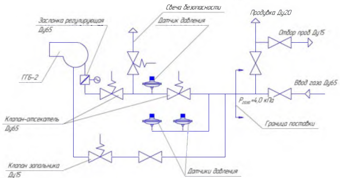
Принципиальная схема подачи газа к котлу с горелкой ГГБ-2 (плавное регулирование) Е-1,6-09ГМН - P_{газа} = 4,0 кПа Е-2,5-0,9ГМН - P_{газа} = 8,0 кПа
